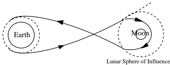
Fig.2 Lunar Free Return Trajectory
